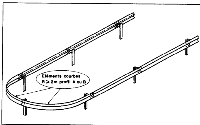
musoir de profil A ou B, de rayon supérieur ou égal à deux mètres.
