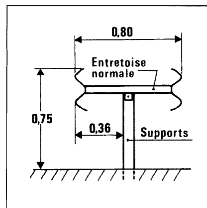
encombrement des glissières doubles.
