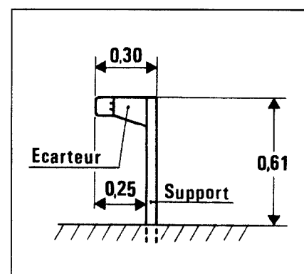
encombrement des glissières simples.
